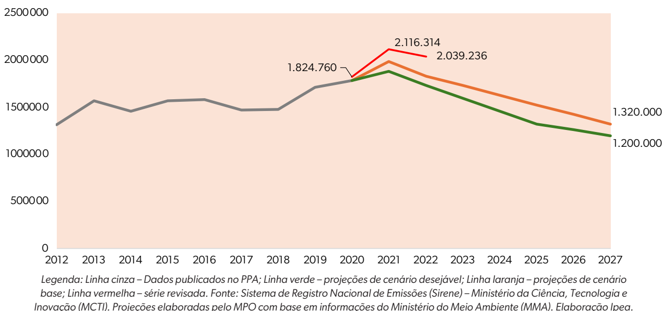
GRÁFICO: EMISSÃO DE GASES DE EFEITO ESTUFA (GEE) NO BRASIL (GWP-AR5) (GG)
