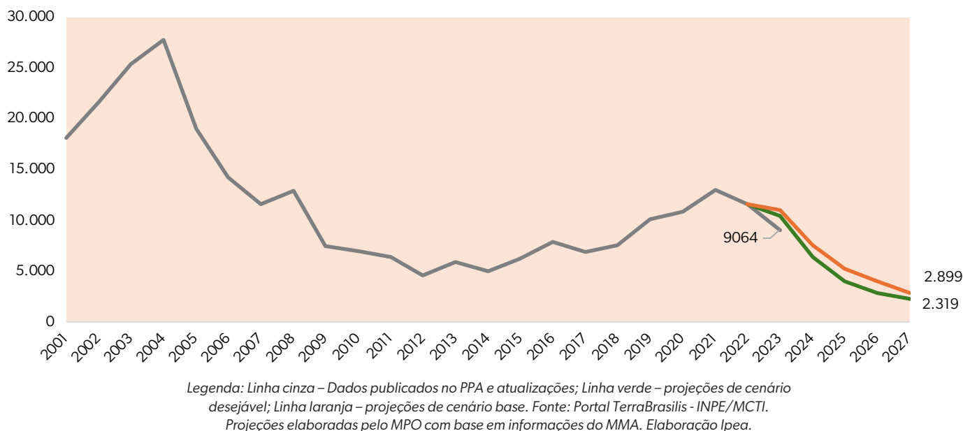
GRÁFICO: DESMATAMENTO ANUAL NO BIOMA AMAZÔNIA (EM KM 2 )
