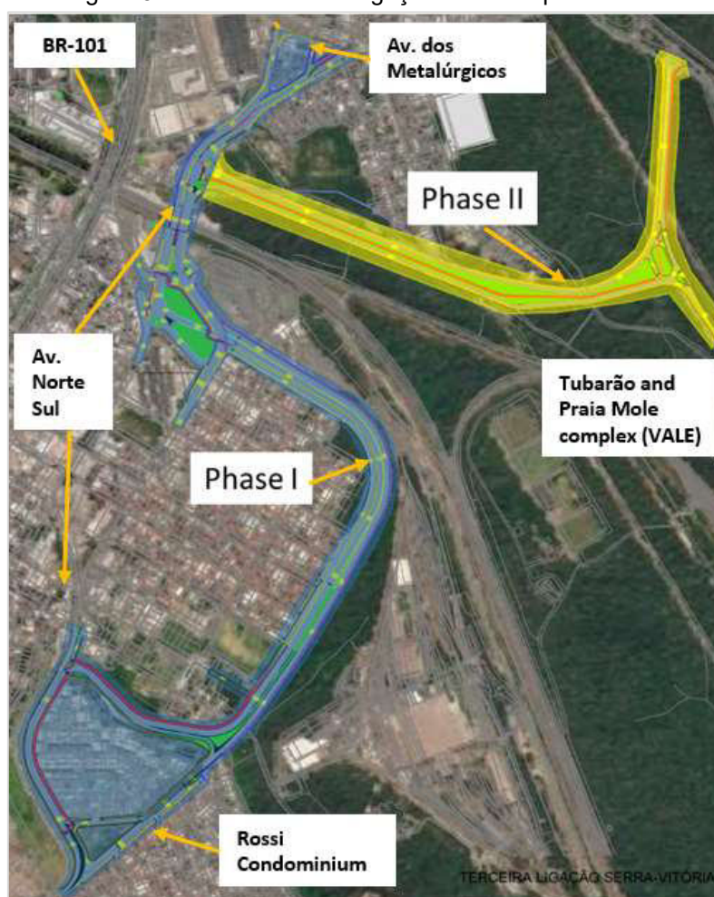
Figura 5 – Terceira Via de Ligação de Serra para Vitória
