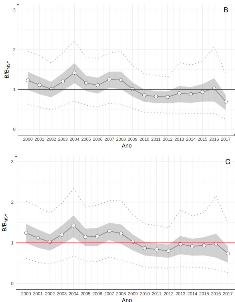
Figura 6: Séries temporais das razões entre biomassas e biomassas sob os rendimentos máximos sustentáveis estimados pelo (A) modelo 0; (B) modelo 2, e; (C) modelo 4. Círculos brancos - estimativas médias; Área sombreada cinza - intervalo de credibilidade de 50%; Linhas tracejadas cinzas - intervalo de credibilidade de 95%.
