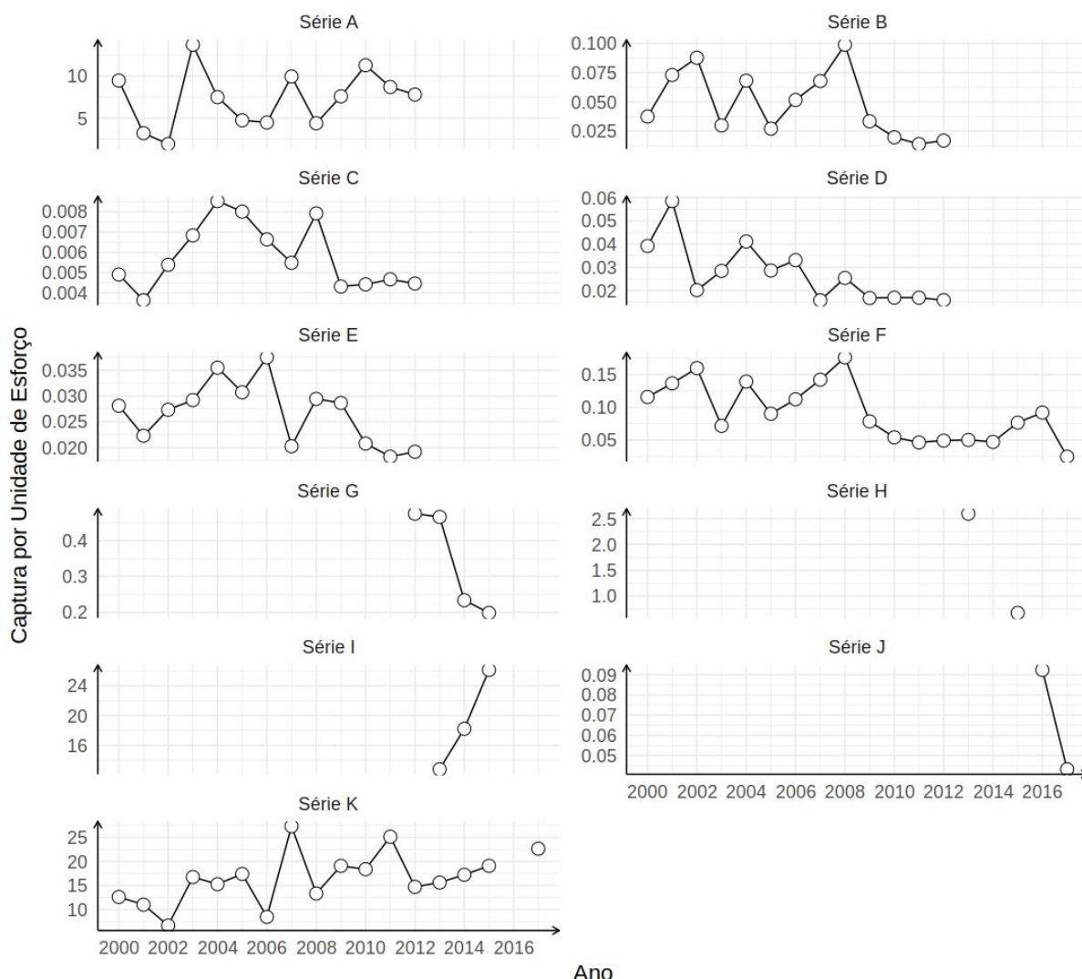
Figura 2: Séries temporais de captura por unidade de esforço de Tainha ( Mugil liza ), estoque Sul, entre os anos de 2000 e 2017. Série A - Pesca industrial de cerco/traineira de Santa Catarina em t/dias de pesca (UNIVALI); Série B - Pesca costeira de São Paulo em t/viagem (IP/SP); Série C - Pesca estuarina de São Paulo em t/viagem (IP/SP); Série D - Pesca costeira de emalha de São Paulo em t/dias de pesca (IP/SP); Série E - Pesca estuarina de emalha de São Paulo em t/dias de pesca (IP/SP); Série F - Pesca artesanal e industrial do estado de São Paulo em t/viagem (IP/SP); Série G - Pesca artesanal do Rio Grande do Sul em t/viagem (FURG/LEA); Série H - Pesca semi-industrial do Rio Grande do Sul em t/viagem (FURG/LEA); Série I - Pesca industrial do Rio Grande do Sul em t/viagem (FURG/LEA); Série J - Pesca de cerco-fixado de São Paulo t/descarga (IP/SP); Série K - Pesca industrial de cerco/traineira de Santa Catarina em t/viagem (UNIVALI).
