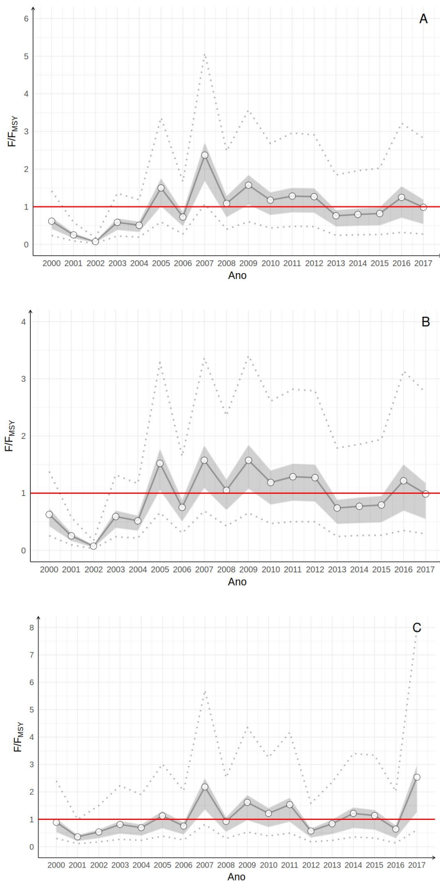
Figura 7: Séries temporais das razões entre taxa de exploração e taxa de exploração sob os rendimentos máximos sustentáveis estimados pelo (A) modelo 0; (B) modelo 2, e; (C) modelo 4.
