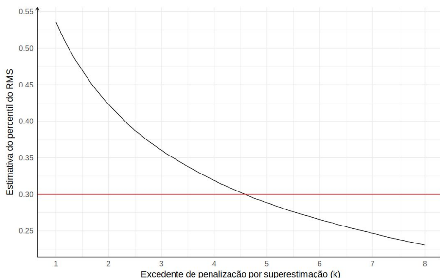
Figura 11: Decaimento da estimativa do percentil do RMS em função do excedente de penalização por superestimação (k) proposto.
