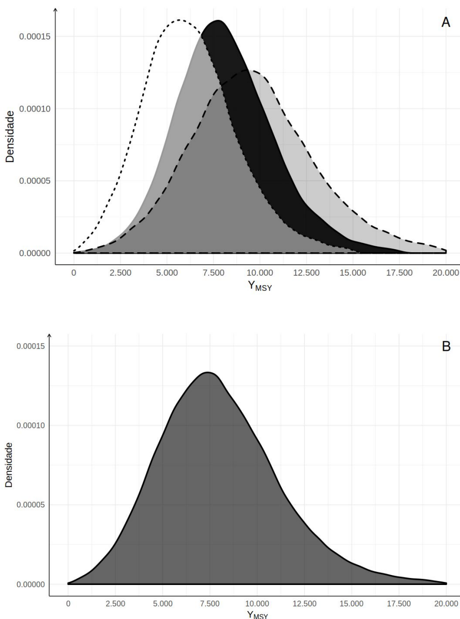
Figura 9: Distribuições posteriores para os rendimentos máximos sustentáveis estimados (A) para cada um dos três modelos ajustados, Modelo 0 - curva cinza e linha tracejada; Modelo 2 - curva preta e linha sólida, e; Modelo 4 - curva branca e linha pontilhada, e; (B) para a distribuição de mistura resultante dos três modelos juntos.
