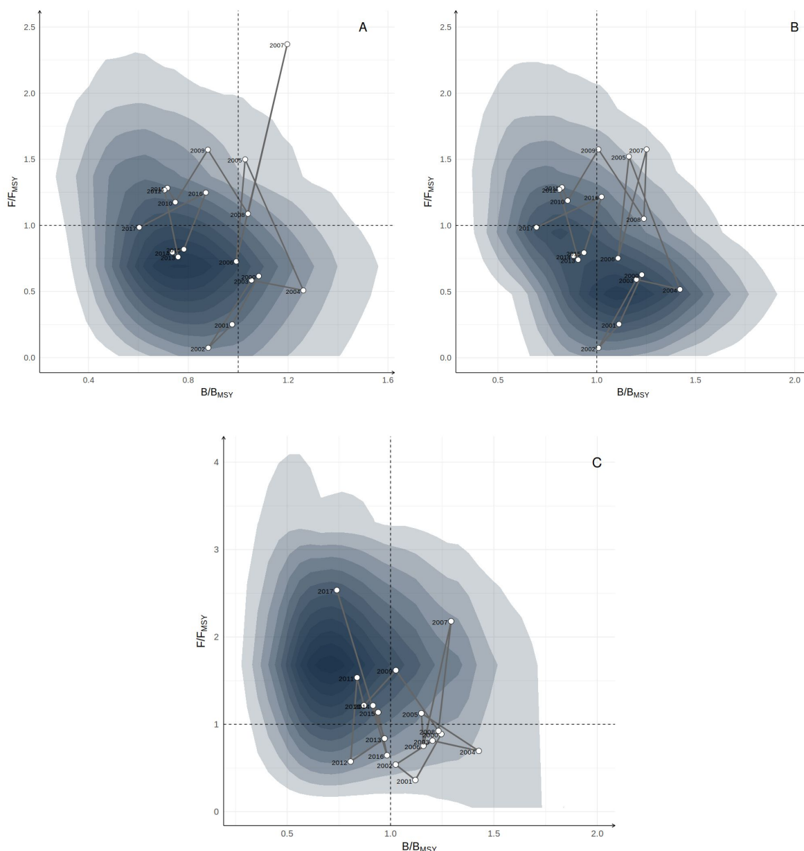
Figura 8: Diagrama de fases ou Kobe plot para Tainha ( Mugil liza ), estoque Sul. (A) Modelo 0; (B) Modelo 2, e; (C) Modelo 4.
