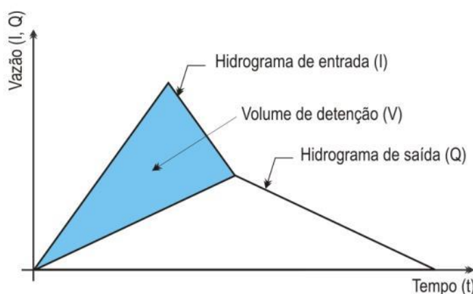
Figura 80. Determinação do volume de retenção: Hidrogramas de entrada e saída.
