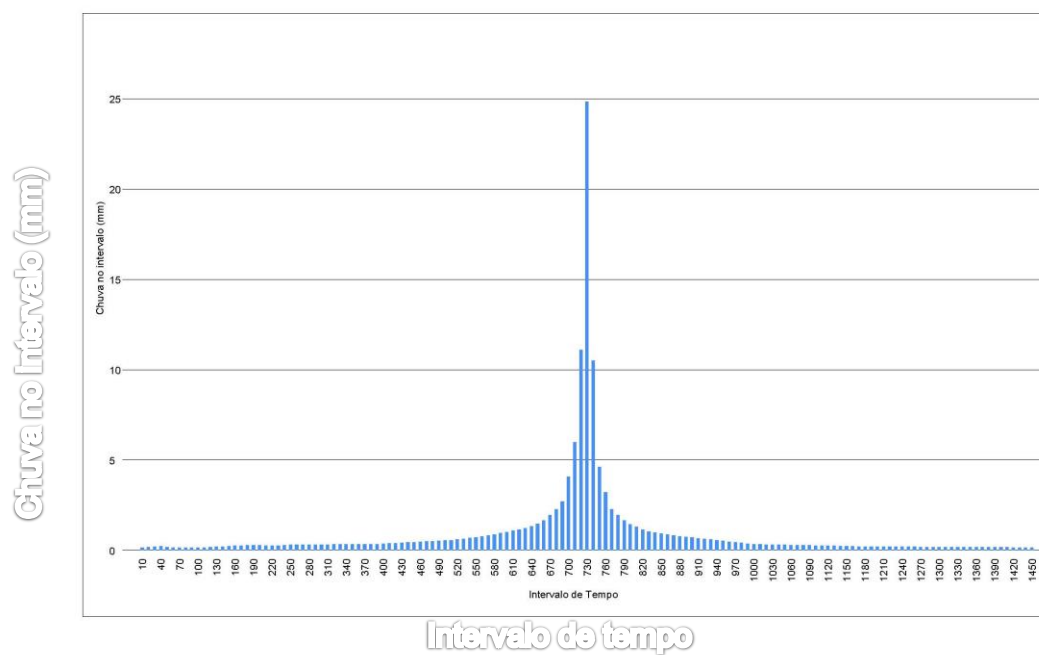
Figura 86 – Hietograma TR 25 anos discrição 10 minutos
