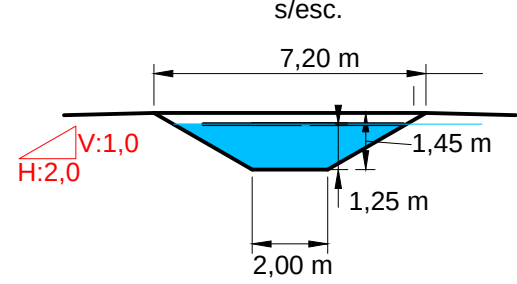
Seção Tipo canal SB-2A
