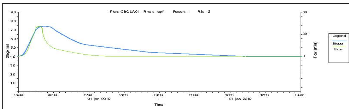
Figura 89 - Hidrograma ponto 2, TR 25 anos, linha em azul: Nível da água [m], linha verde vazão [m³/s].
