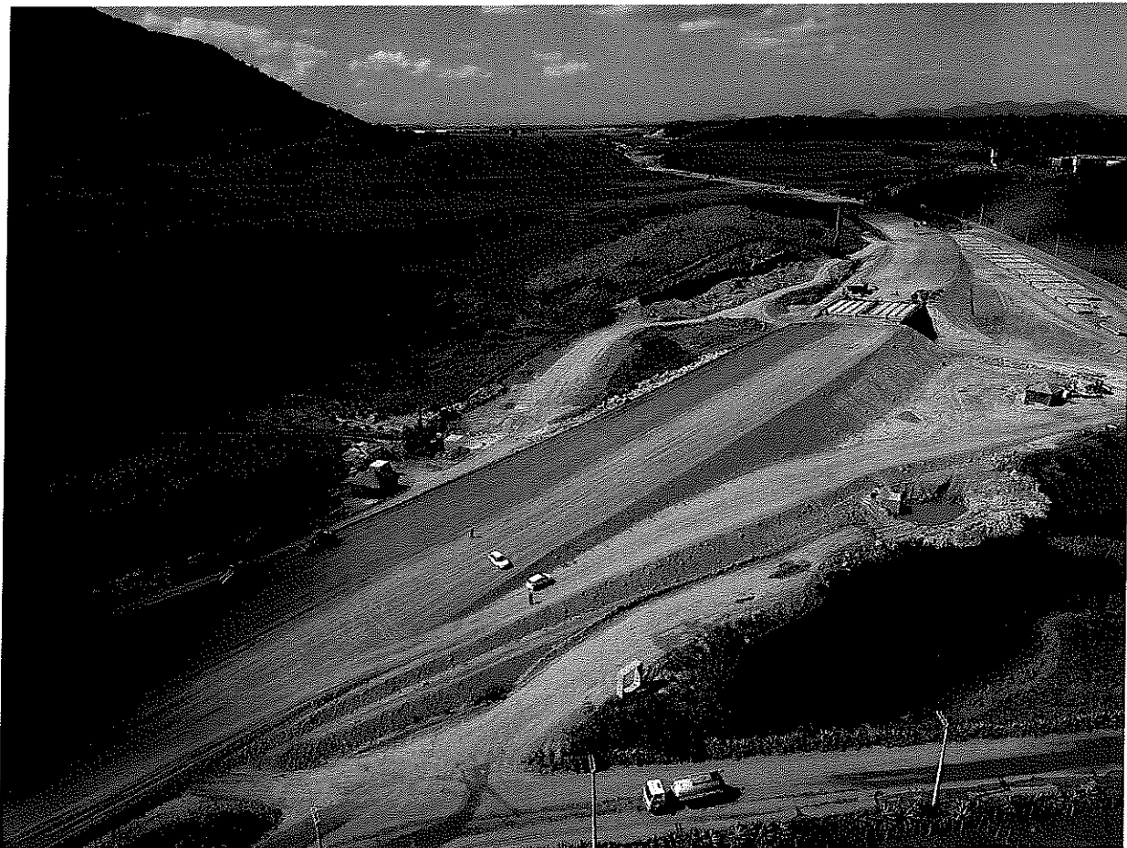
Foto 02 – Vista geral da estaca 320 (terraplenagem em estágio avançado, preparando para início da pavimentação).
