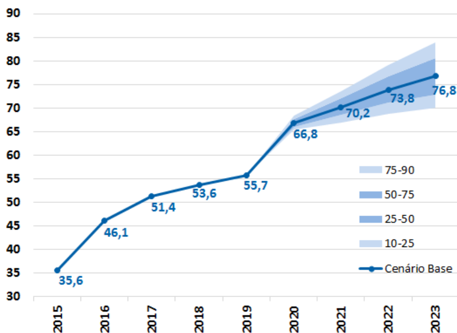
Figura 9 - Cenários Estocásticos para DLSP/PIB: Cenário Base
