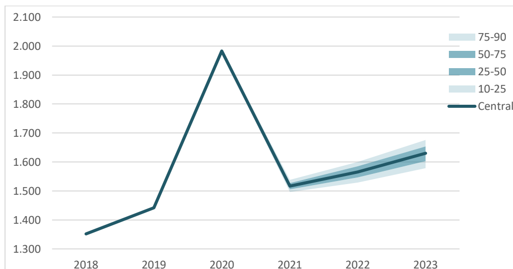
Figura 6 - Espectro de cenários alternativos para Despesas Totais (R$ bilhões)
