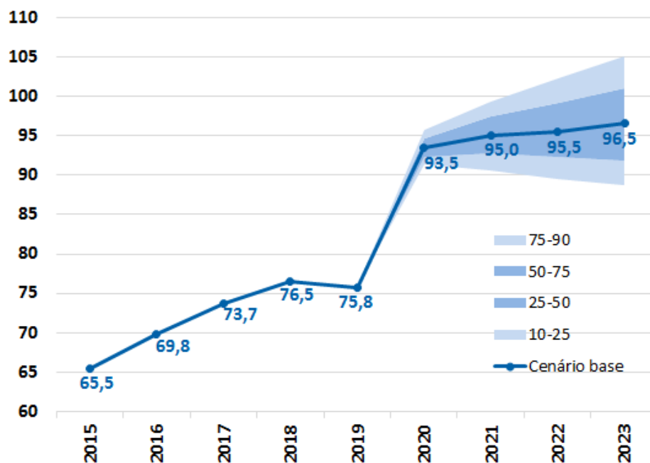
Figura 8 - Cenários Estocásticos para DBGG/PIB: Cenário Base
