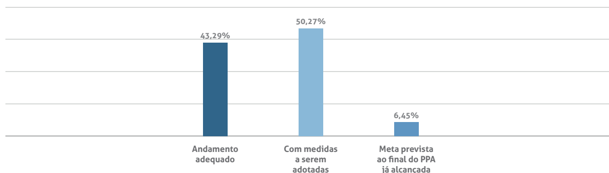
Gráfico 10 - Desempenho das Metas do PPA acumulado até 2017
