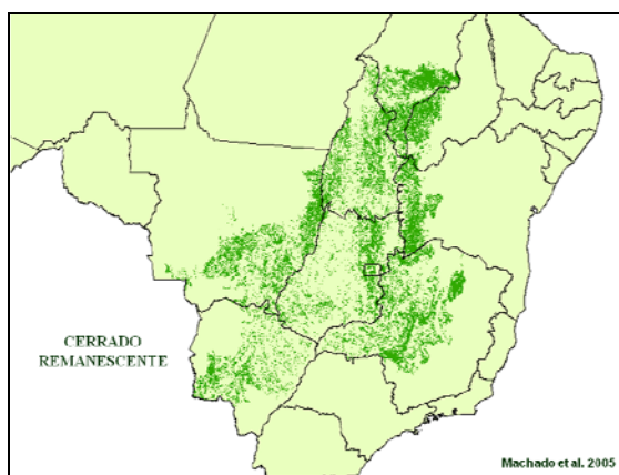
Figura 24 – Cobertura remanescente de Cerrado
