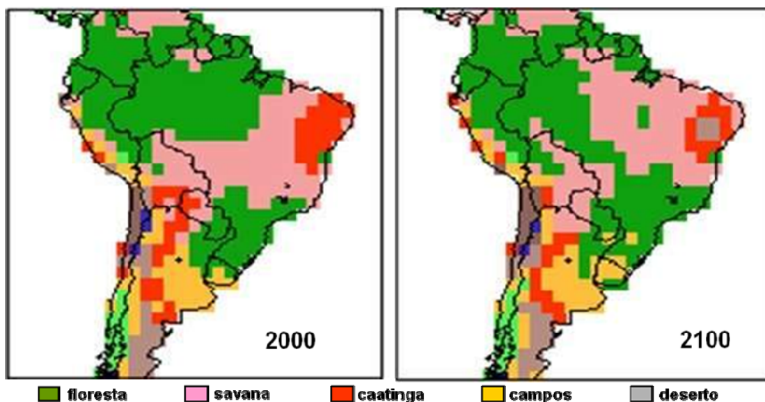
Figura 4 – Alterações previstas nos ecossistemas brasileiros Fontes: Oyama & Nobre, 2003 e Salazar, Oyama & Nobre, 2007
