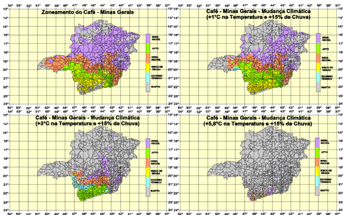
Figura 22 – Café Arábica em Minas Gerais – simulação para os vários cenários do IPCC (aumento de 15% nas chuvas e de 1ºC, 3ºC e 5,8ºC.)
