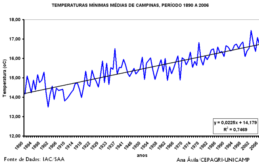
Figura 5 – Temperaturas mínimas médias em Campinas – período 1890 a 2006.
