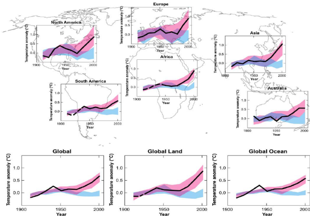
Figura 3. Comparação das mudanças observadas de escalas continental – e global – na temperatura da superfície com resultados simulados por modelos climáticos, usando-se forçamentos naturais e antrópicos. As médias decenais das observações são apresentadas para o período de 1906 a 2005 (linha preta) plotadas sobre o centro da década e relativas à média correspondente para 1901-1950. As linhas são tracejadas quando a cobertura espacial é inferior a 50%. As zonas azuis indicam a faixa de 5 a 95% para as 19 simulações dos 5 modelos climáticos com o uso apenas dos forçamentos naturais devidos à atividade solar e aos vulcões. As zonas vermelhas mostram a faixa de 5 a 95% para as 58 simulações dos 14 modelos climáticos com o uso dos forçamentos natural e antrópico.
