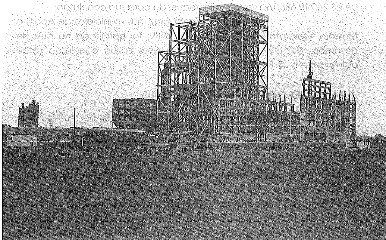
Usina termelétrica de Jacuí - RS
