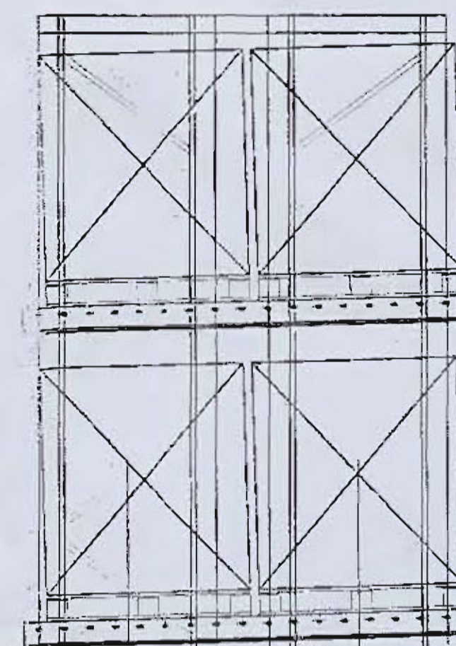
ESTRUTURA FLOW- TRACK/ELEVAÇÃO LATERAL-TIPO
