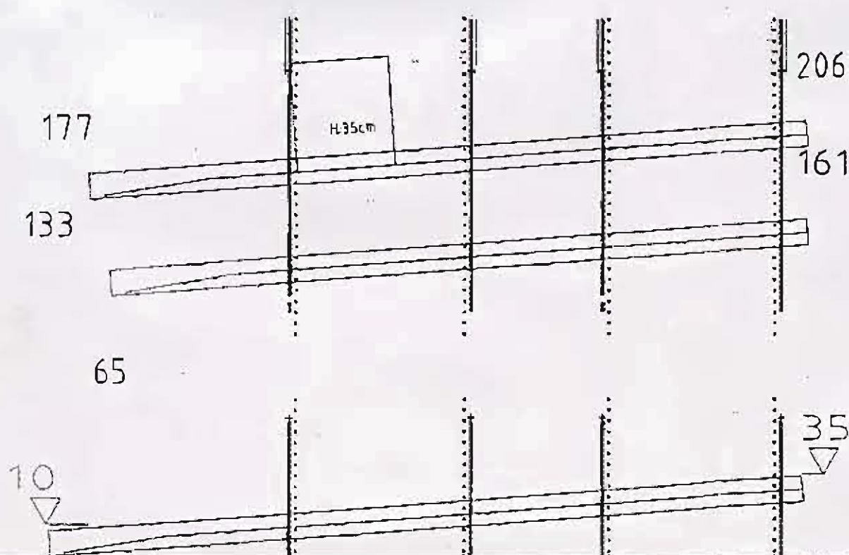
FLOW-RACK/ELEVAÇÃO LATERAL-TIPO FULL CASE(CORTE B-B)
