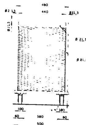
VISTA FRONTAL ESC. 1:10
