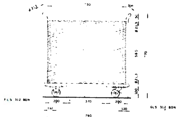
VISTA LATERAL ESC 1:10
