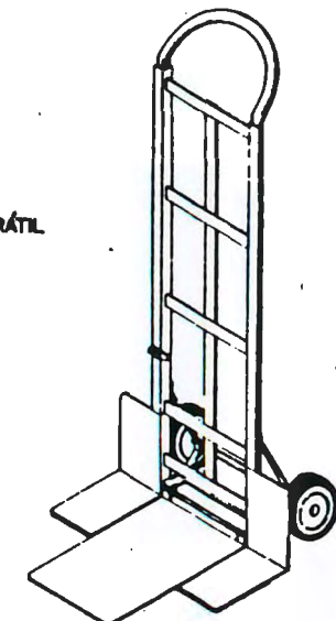
PERSPECTIVA ESC. 1:10
