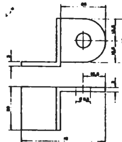
DOBRADILHA DA PLAT. RETRÁTIL ESC. 1:1
