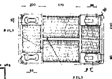
VISTA INFERIOR ESC 1:10
