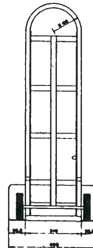
VISTA POSTERIOR ESC. 1:10
