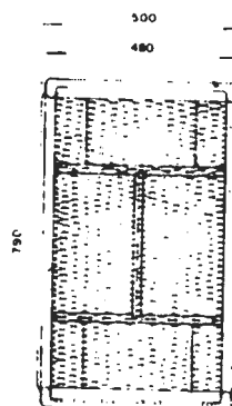
VISTA SUPERIOR ESC 1:10
