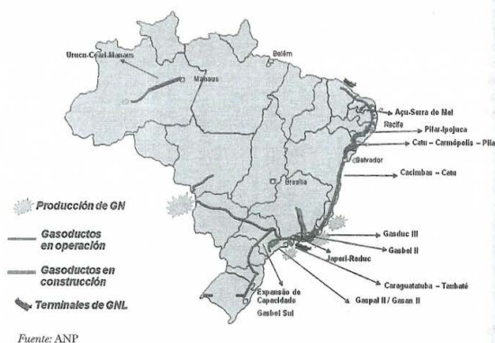
MAPA 4.—Infraestructura de transporte de gas natural en Brasil en 2010
