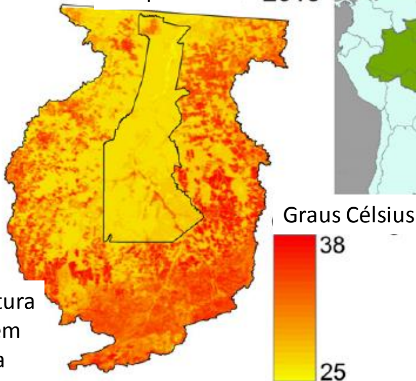
Temperatura - 2010
