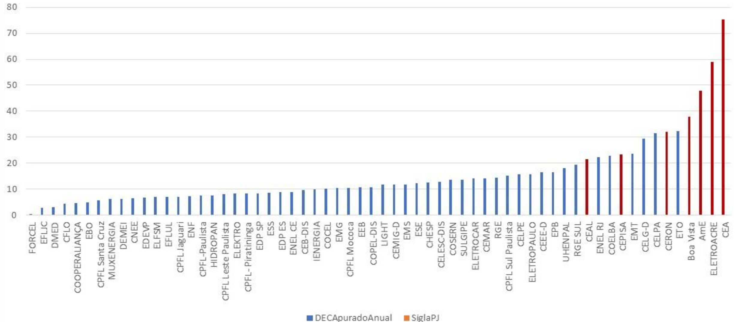
Duração Média das Interrupções (DEC 2016)
