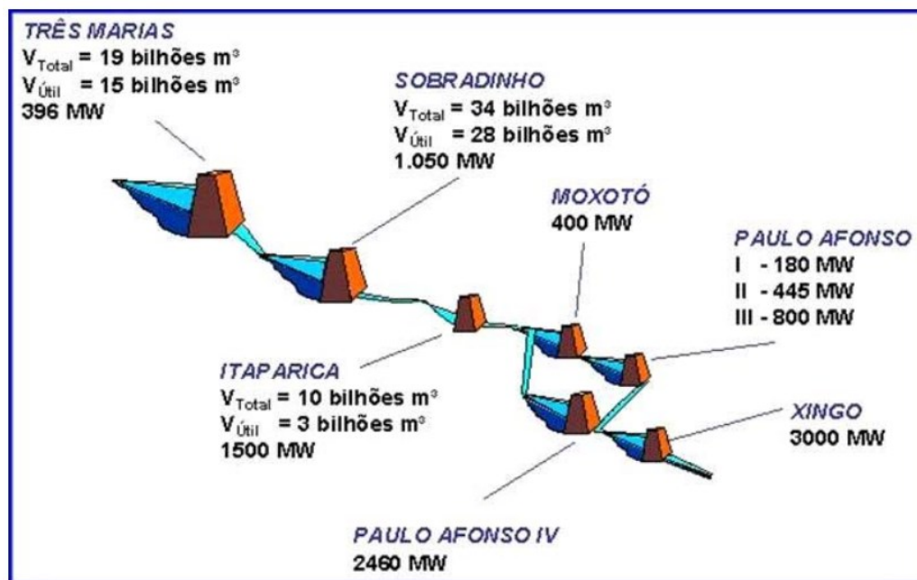
Figura 2 – Reservatórios da bacia do São Francisco 5
