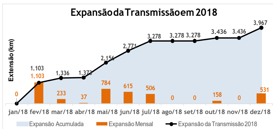
Figura 002 - Indicador - Previsão Expansão da Transmissão
