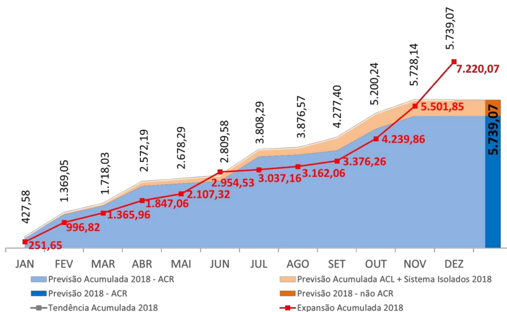
Figura 001 – Indicador - Previsão da Expansão da Geração
